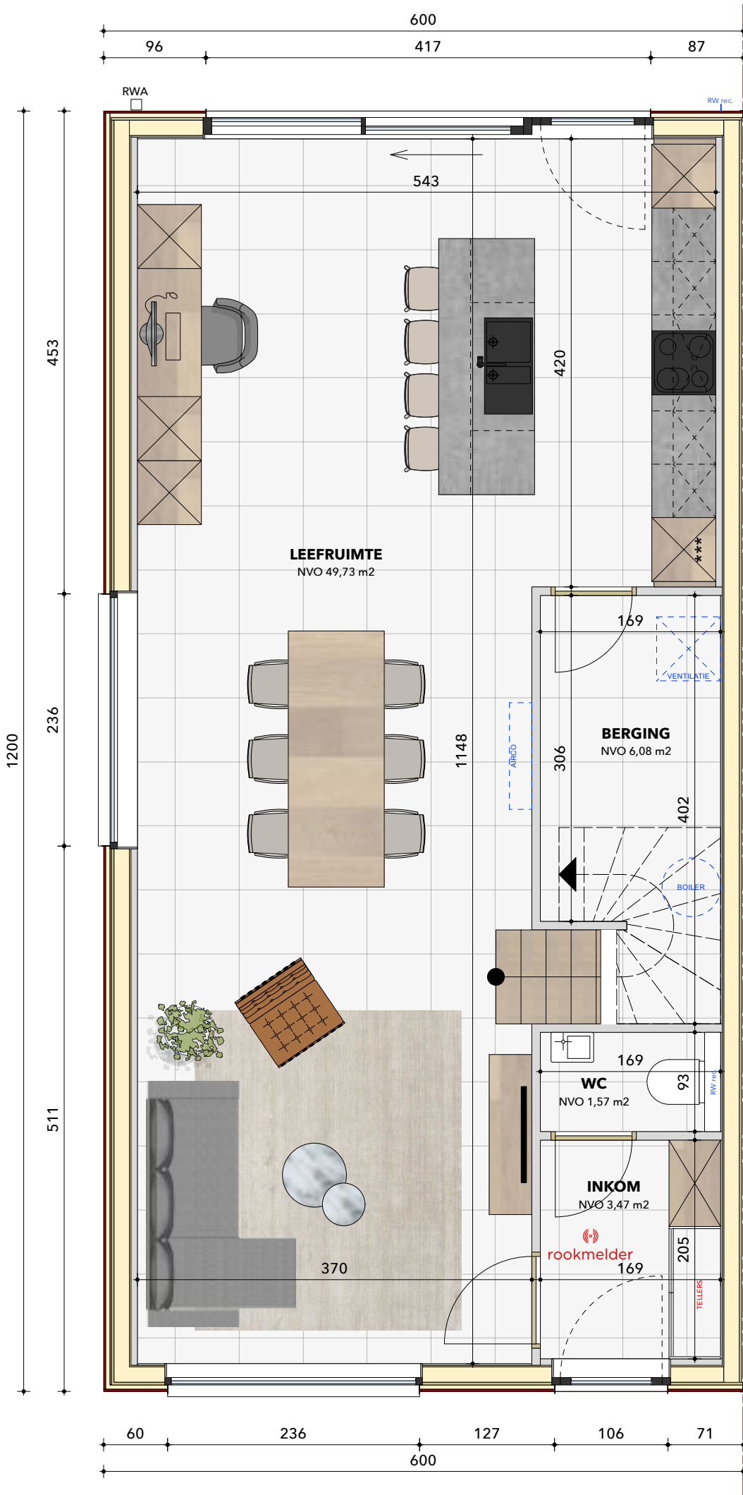
Gelijkvloers
