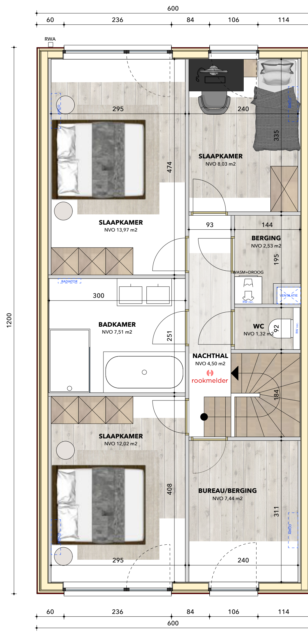
Verdieping
